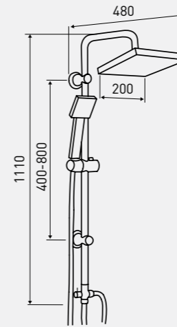
DENIS 60 BL / 63 BL/G
